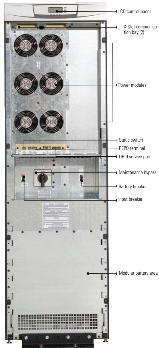
20/30 kVA UPS
